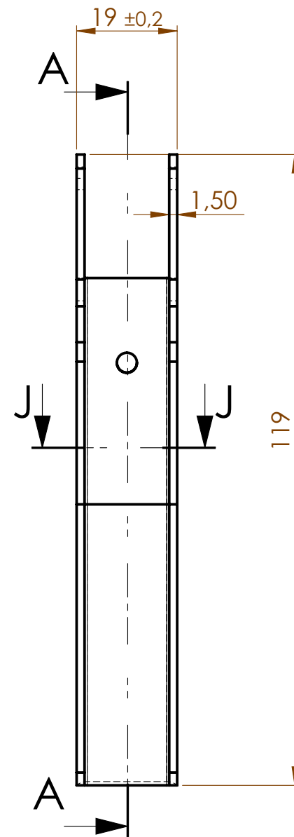
PRZEKRÓJ J-J
